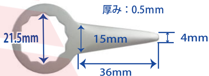
JTC3830C 替刃ショート
