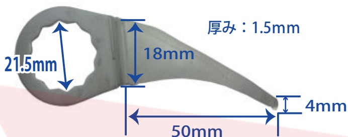
JTC3830A 替刃カーブ
