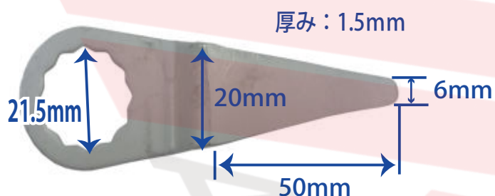
JTC3830B 替刃ストレート
