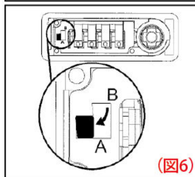
工具箱内部のダイヤル&キーロック部分のリセットレバー
