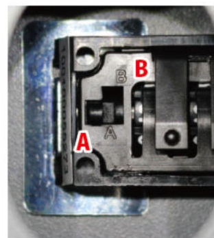
工具箱内部のダイヤル&キーロック部分のリセットレバー
